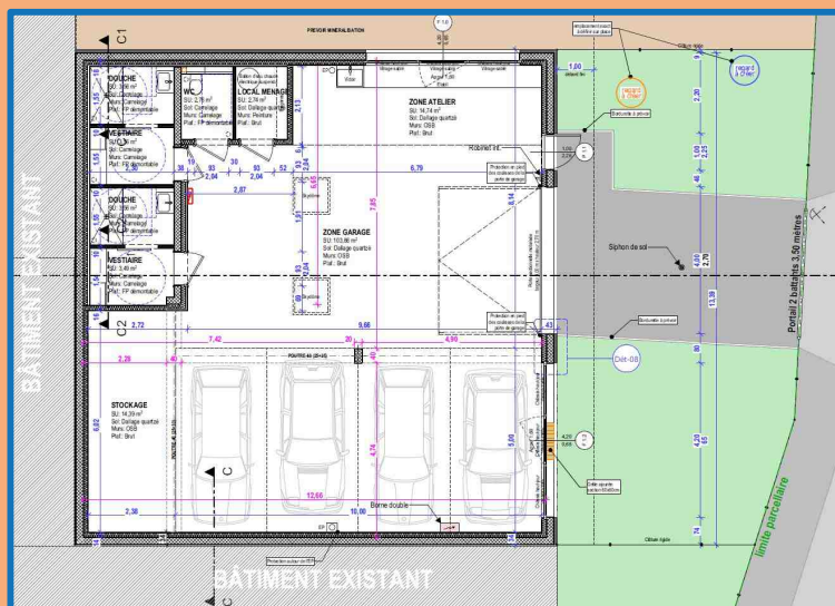
Plan d'intérieur du nouvel atelier communal
